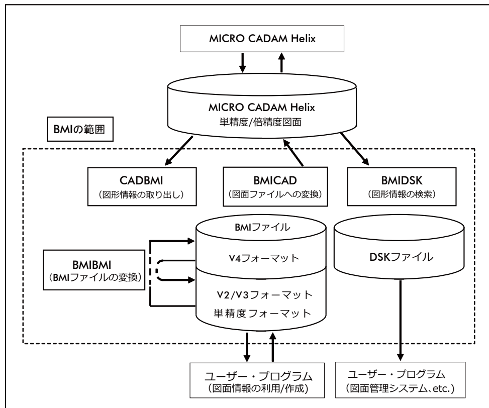
BMIにおける処理概要
