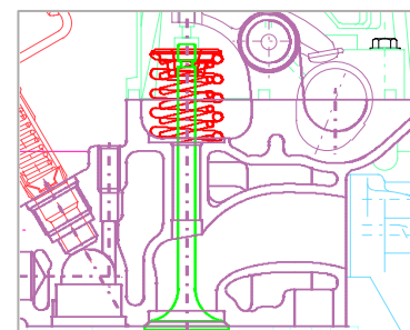
子図 # 4 の編集終了
